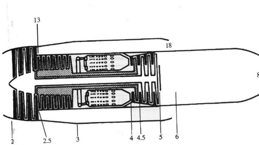
Fig. 3.10 Turbofan a flussi separati
